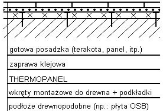
c) przekrój podłogi na podłożu drewnopodobnym
