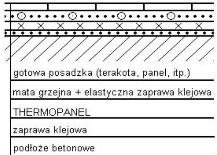
b) przekrój podłogi z ogrzewaniem podłogowym na podłożu betonowym
